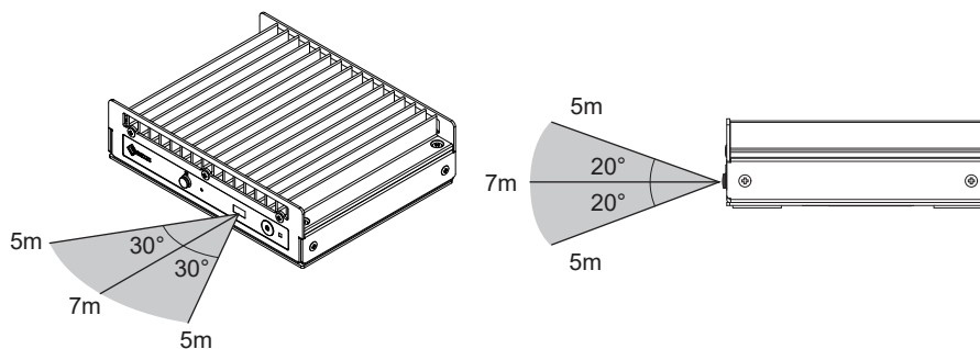
リモコン受光ユニット
