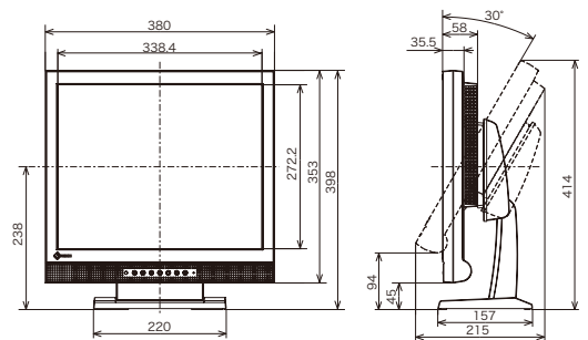
■寸法図 (単位: mm)
