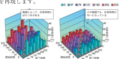
■オーバードライブ回路がない場合 ■オーバードライブ回路がある場合 動画像の輪郭のボヤケを応答時間として評価したグラフです(当社測定値)。この測定方法では、より人間の視覚に近い評価が可能です。
